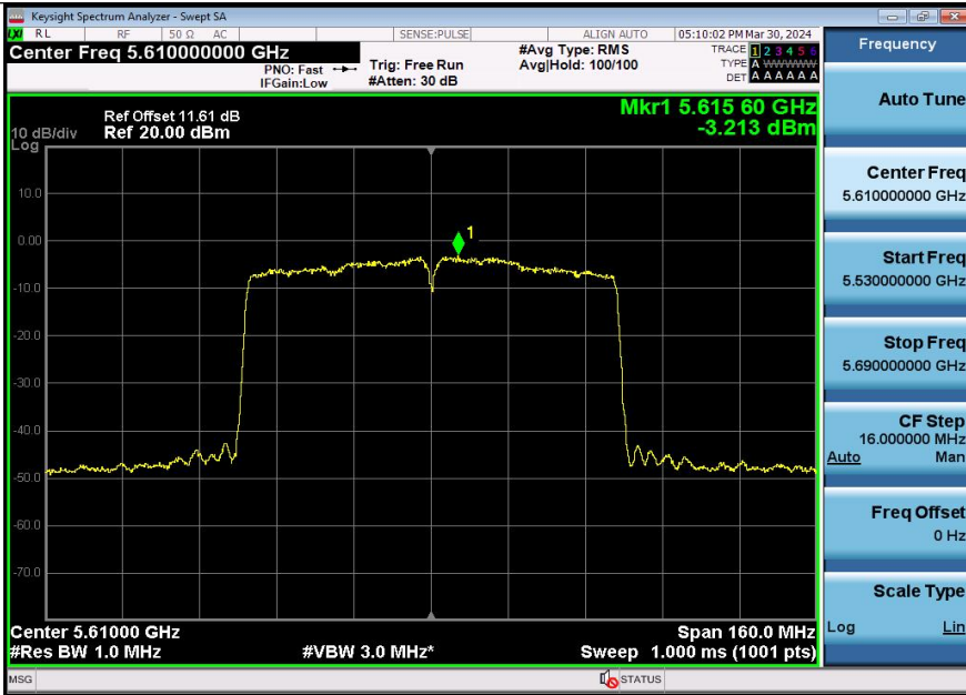
11AX80SISO-Ant2-5610-PASS
