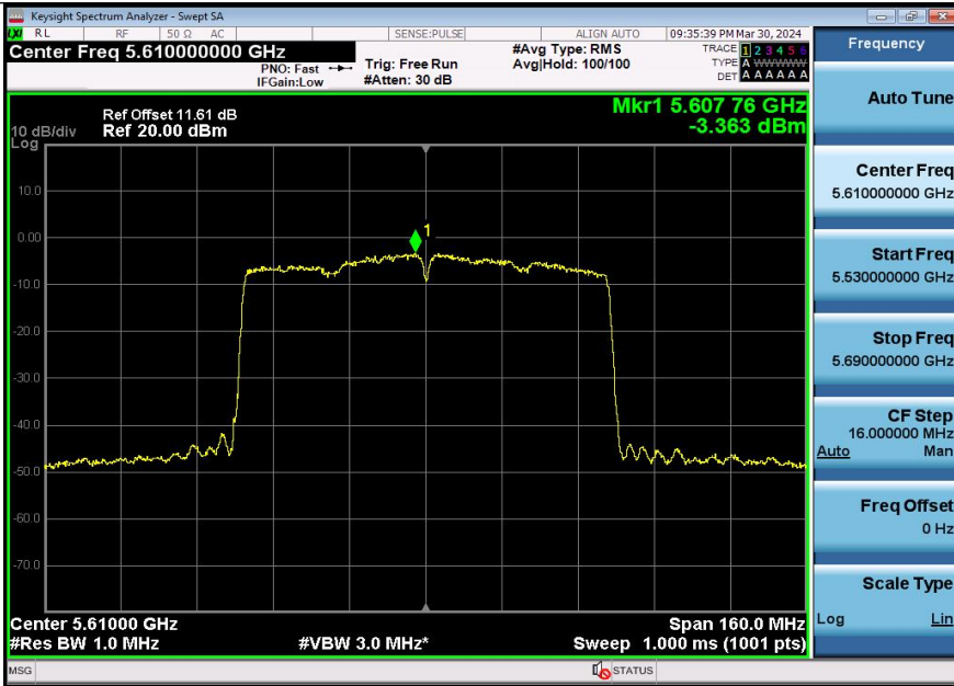
11AX80SISO-Ant1-5610-PASS
