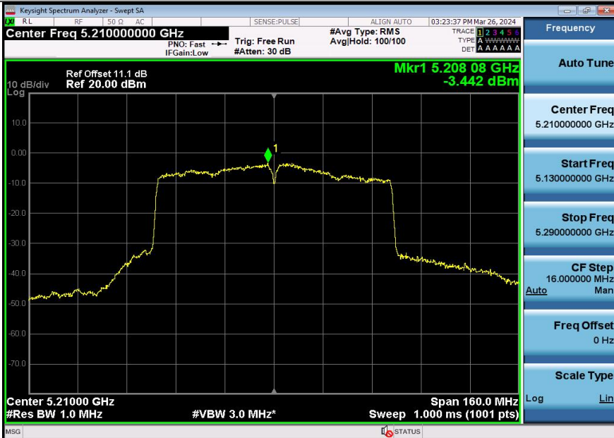
11AX80SISO-Ant1-5210-PASS
