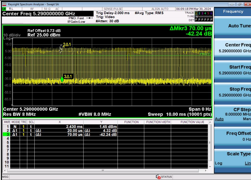
NTNV-11AC80SISO-Ant3-5290
