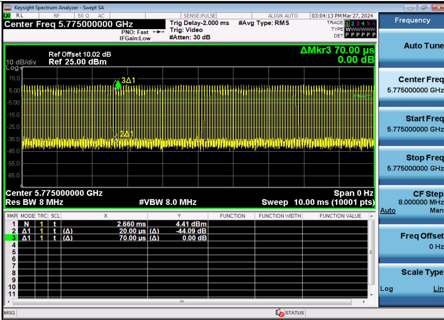
NTNV-11AC80SISO-Ant3-5775
