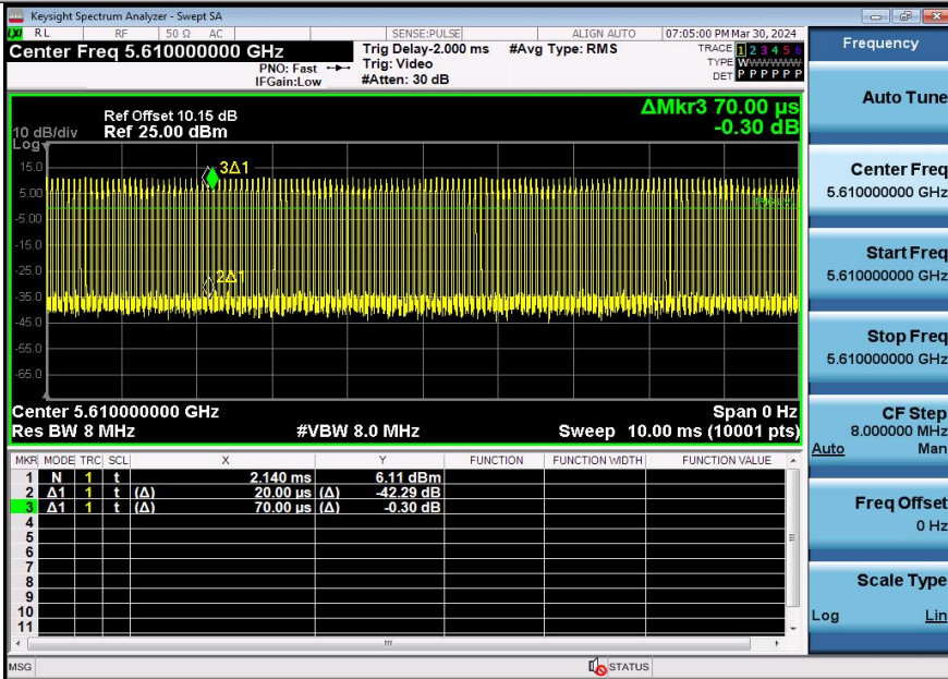
NTNV-11AC80SISO-Ant3-5610
