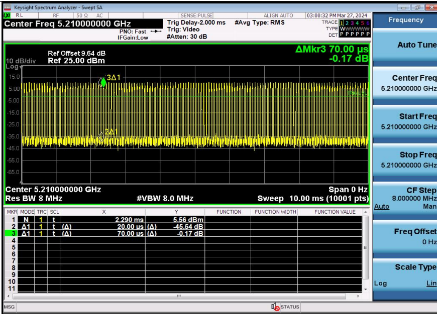
NTNV-11AC80SISO-Ant3-5210
