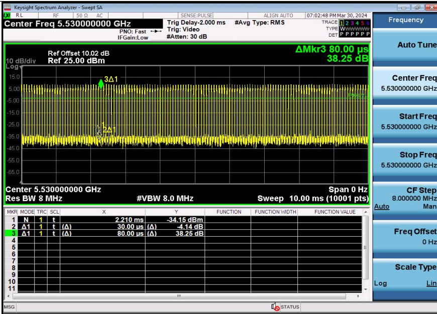
NTNV-11AC80SISO-Ant3-5530
