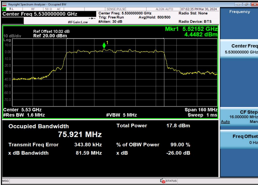
11AC80SISO-Ant3-5530
