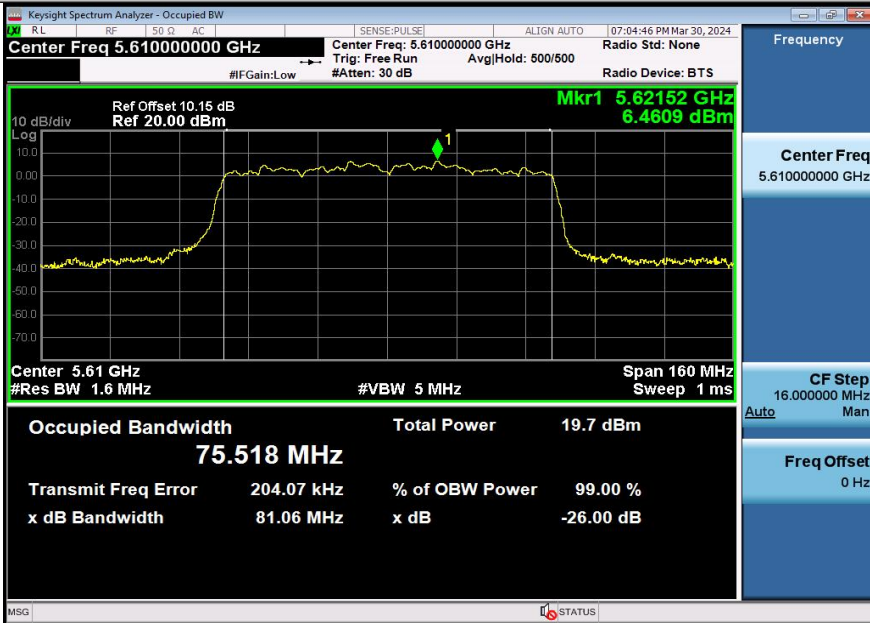
11AC80SISO-Ant3-5610
