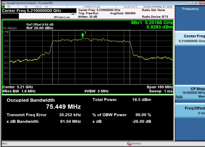
11AC80SISO-Ant3-5210
