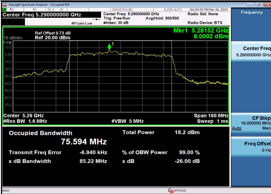
11AC80SISO-Ant3-5290
