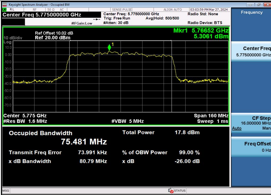
11AC80SISO-Ant3-5775
