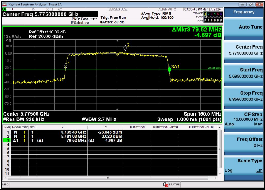
11AX80SISO-Ant3-5775
