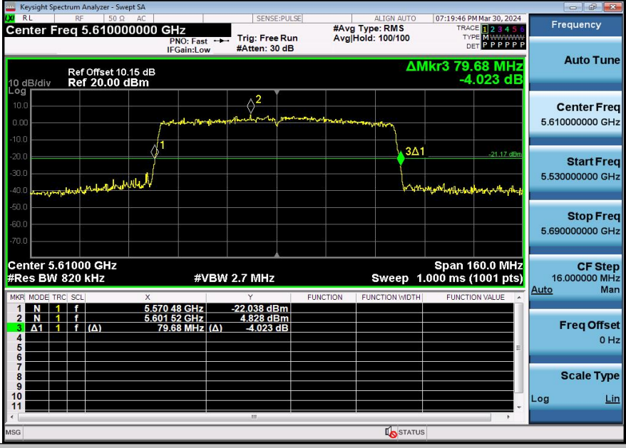
11AX80SISO-Ant3-5610
