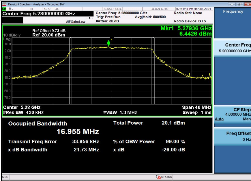
11A-Ant1-5280
