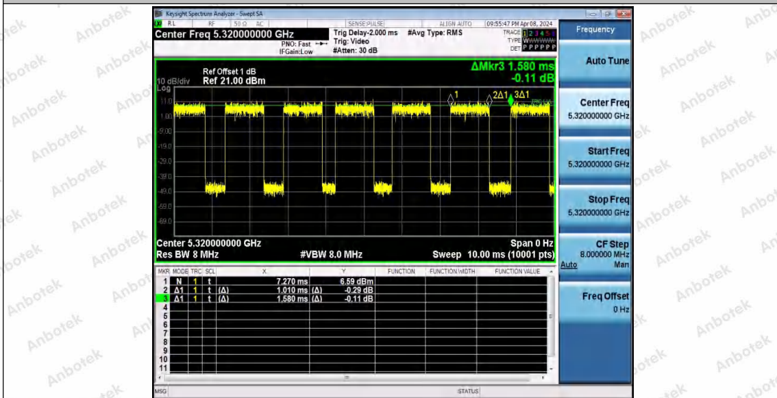
11AX20MIMO_Ant2_5320
