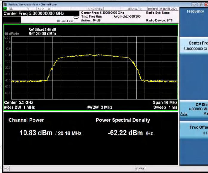
11N20MIMO_Ant2_5300
