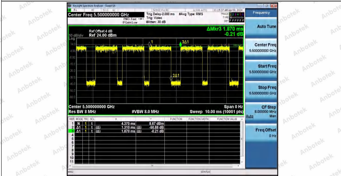
11AC20MIMO_Ant2_5500
