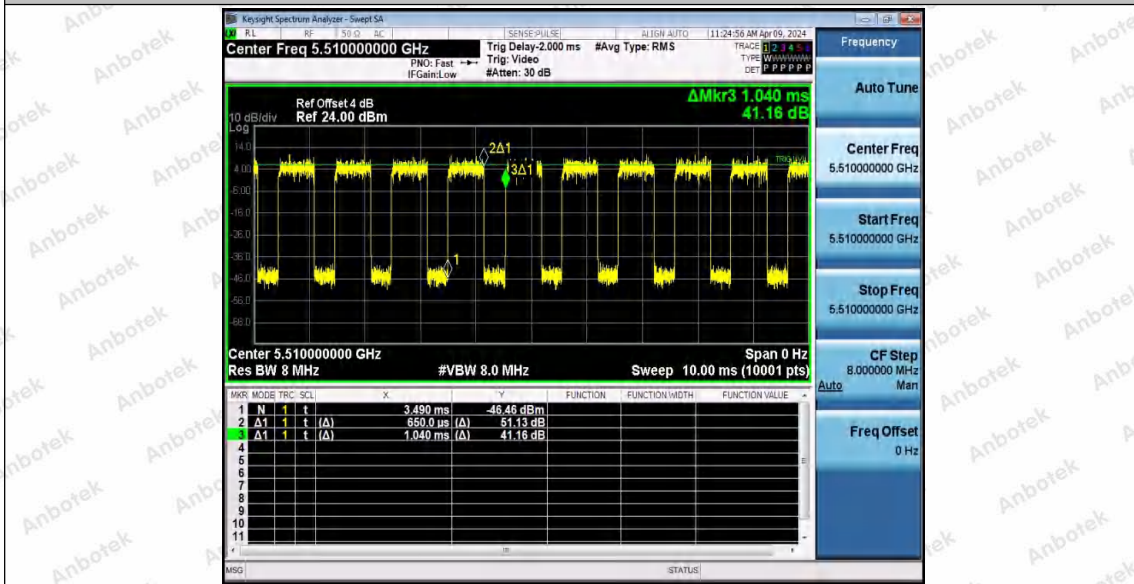
11AC40MIMO_Ant2_5510
