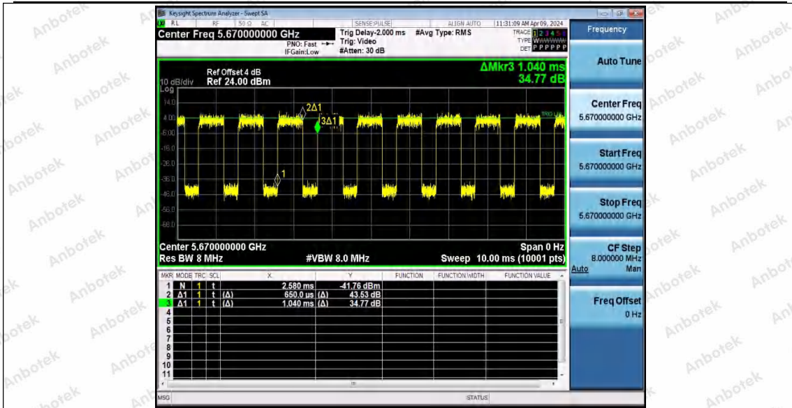
11AC40MIMO_Ant2_5670
