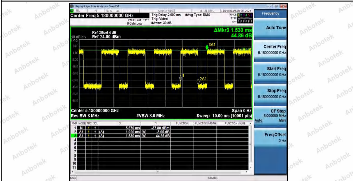
11AX20MIMO_Ant2_5180
