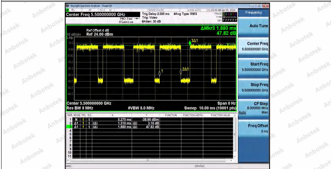
11AC20MIMO_Ant2_5500
