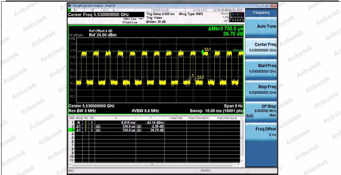
11AC80MIMO_Ant2_5530
