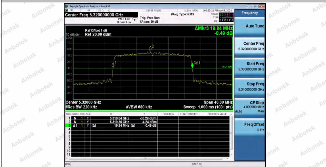
11AX20MIMO_Ant2_5320
