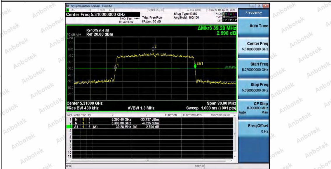
11AX40MIMO_Ant2_5310
