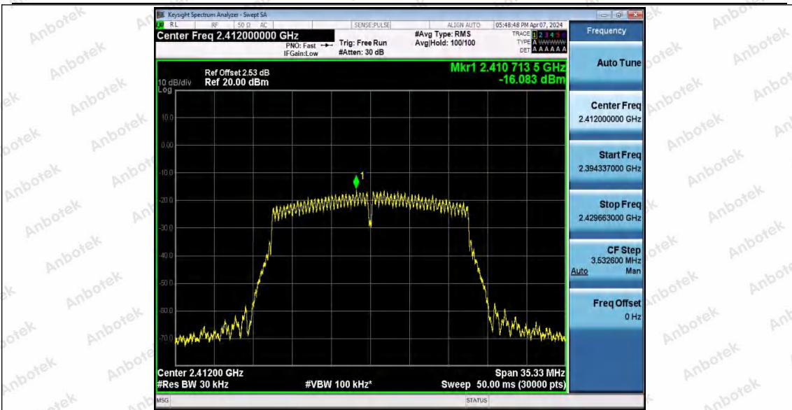
11N20SISO_Ant2_2412
