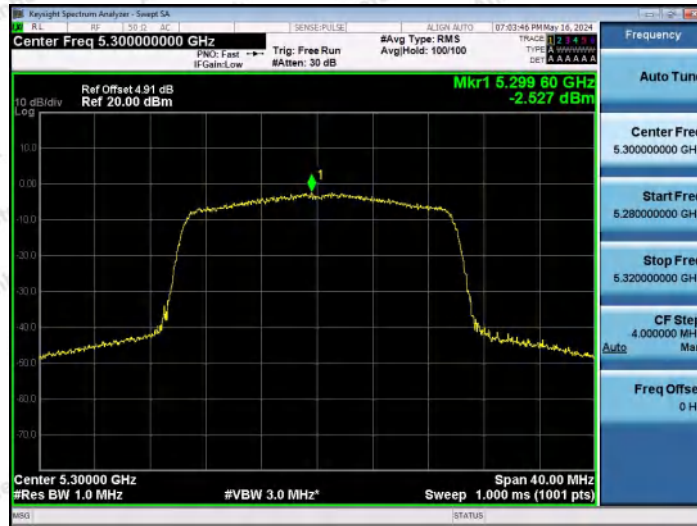
11AX20MIMO-Ant1-5300-PASS
