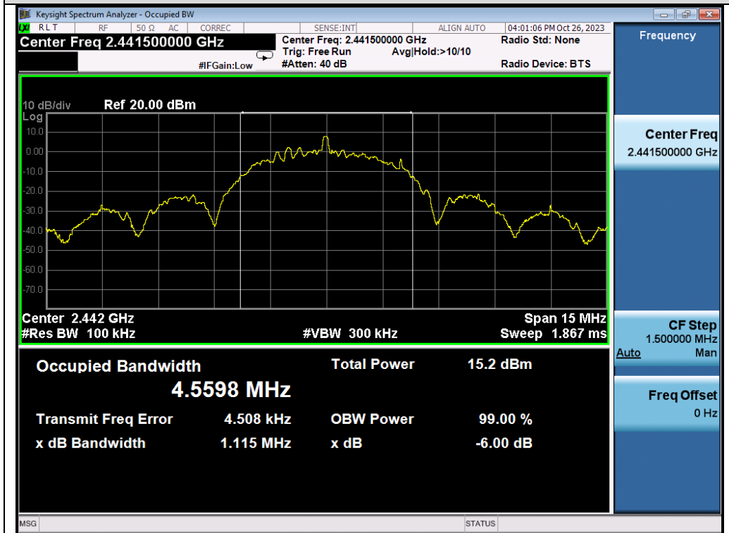
Test_Graph_GFSK_ANT1_2441.5_DTSBW
