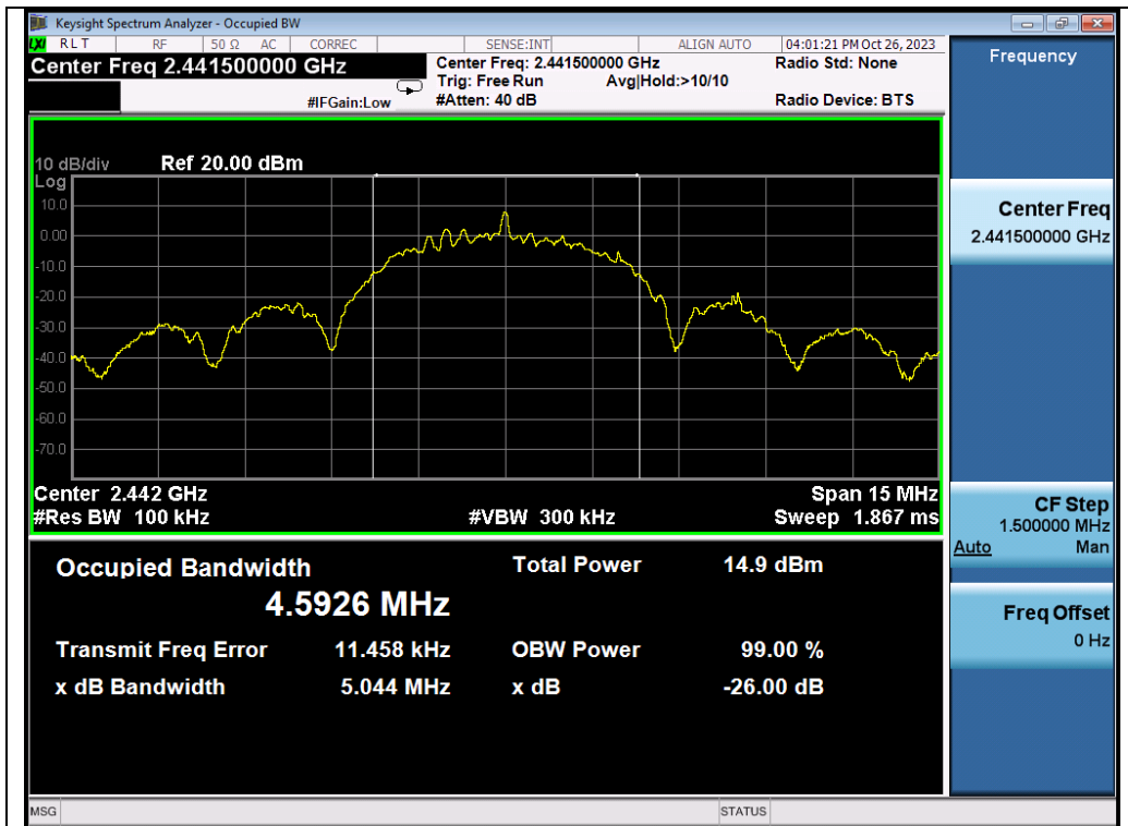
Test_Graph_GFSK_ANT1_2441.5_OBW
