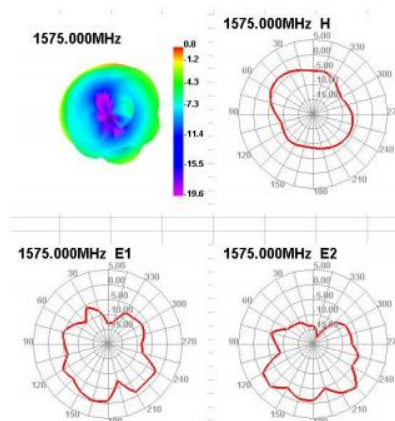
1500.00MHz - 1600.00MHz Gain
