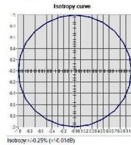
Isotropy: \pm 0.25\% ( \pm 0.01 dB)
