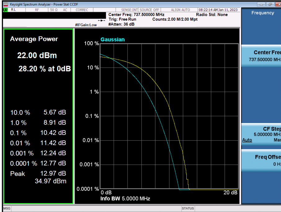
Plot 7-51. PAR Plot (LTE Band 12- 5MHz QPSK - Full RB)
