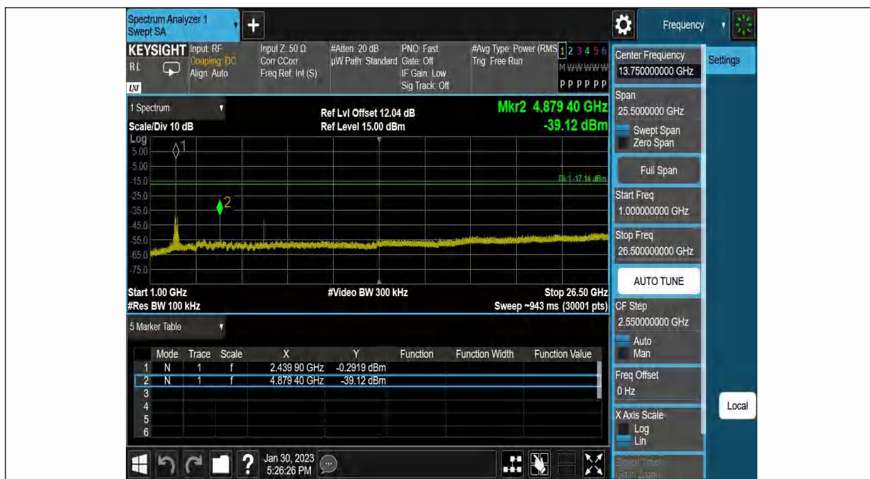
BLE 2M-Ant1-2440-1000~26500-2.86
