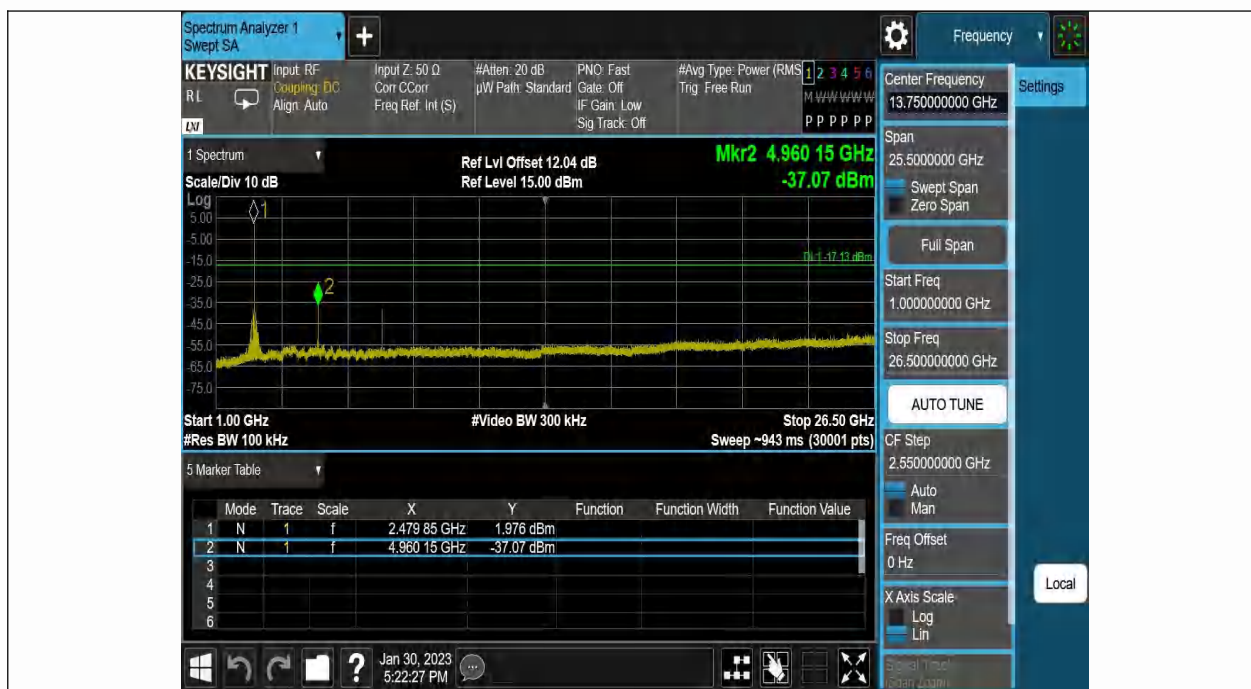
BLE 1M-Ant1-2480-1000~26500-2.87
