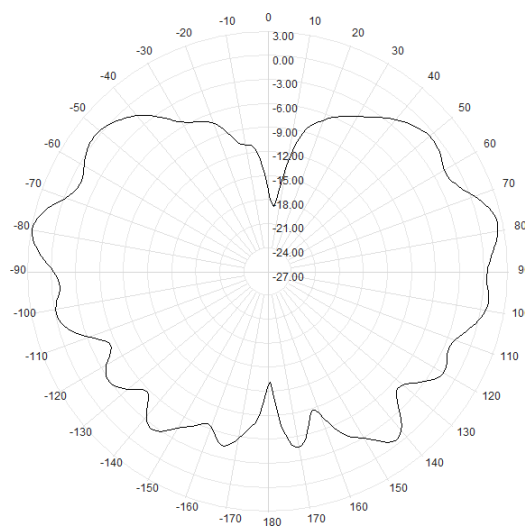
E(890MHz)
