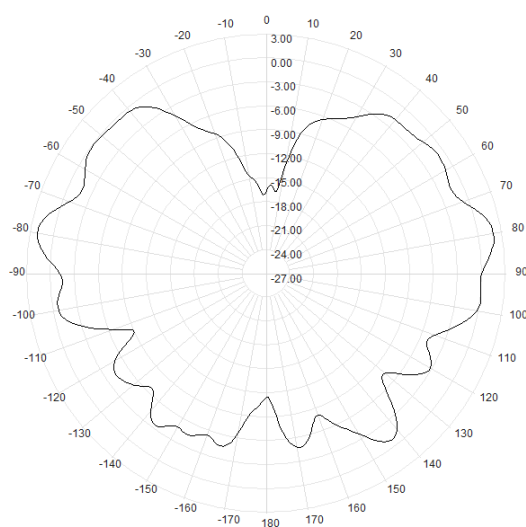
E(850MHz)
