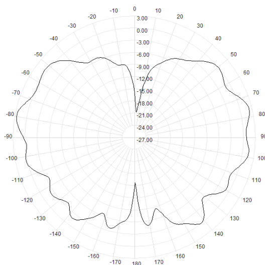
E(930MHz)
