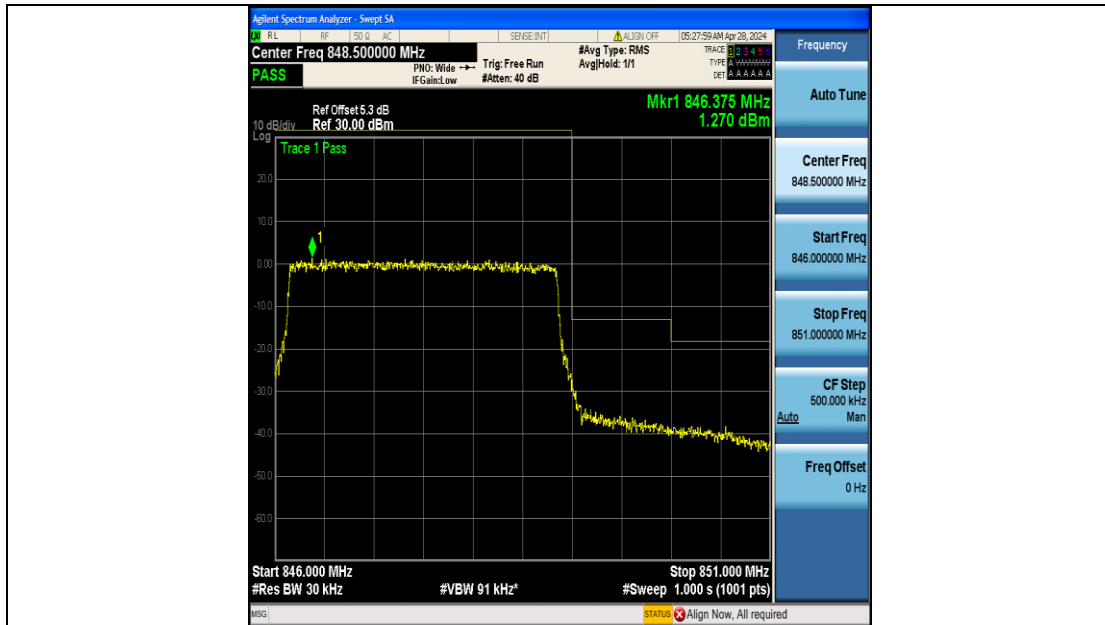
Band5_3MHz_16QAM_20635_15RB#0
