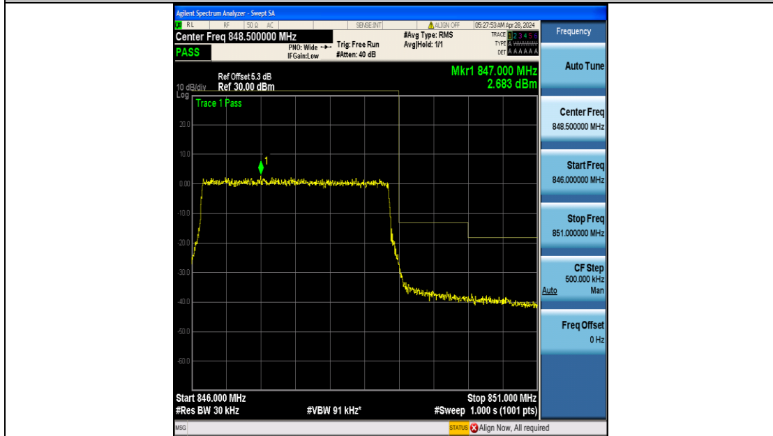
Band5_3MHz_QPSK_20635_15RB#0
