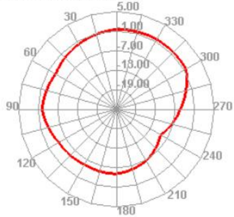
2400.000MHz H
