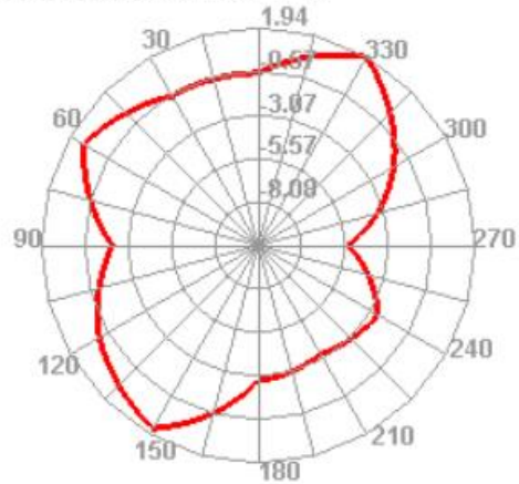
2400.000MHz E2
