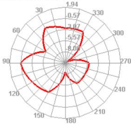
2400.000MHz E1
