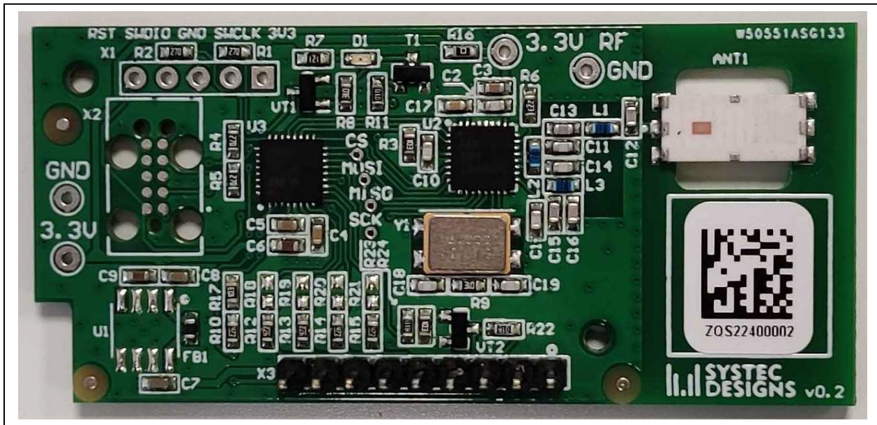
PCB 925 MHz CA3Q Bottom
