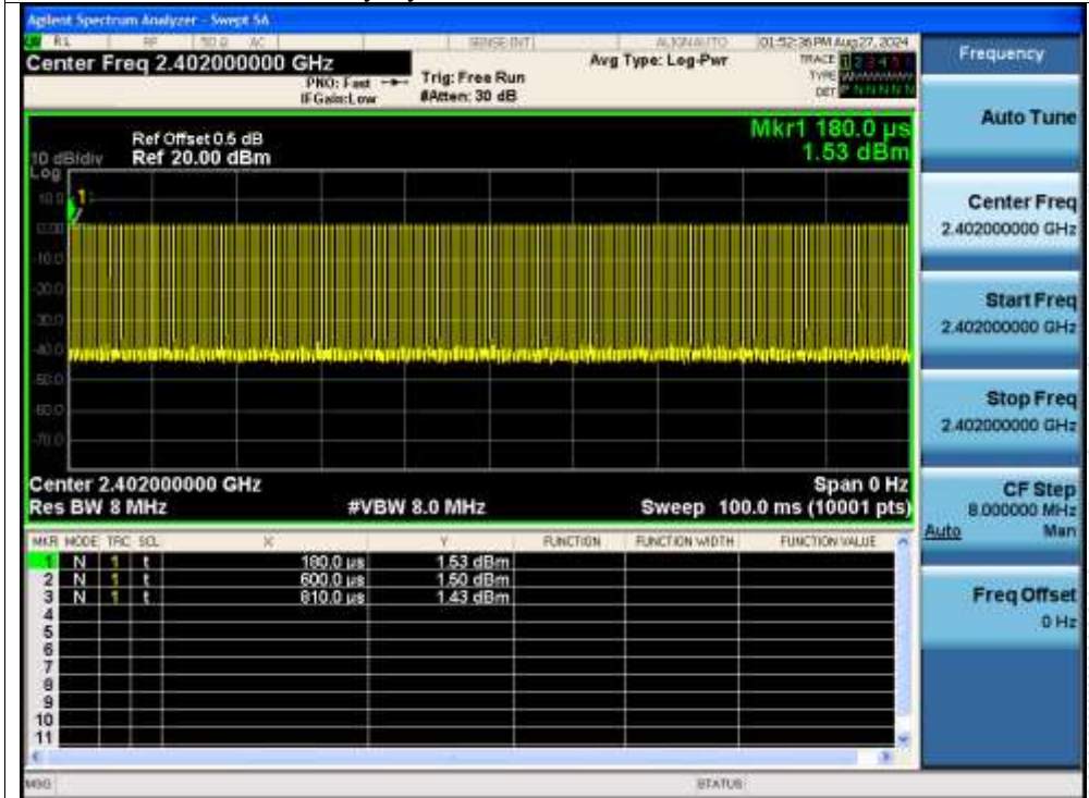
Duty Cycle NVNT BLE 2M 2402MHz
