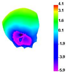
5000.000MHz
