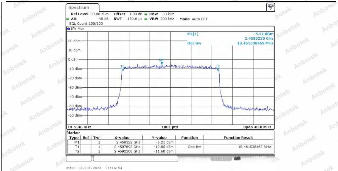
20M_Ant2_2460
