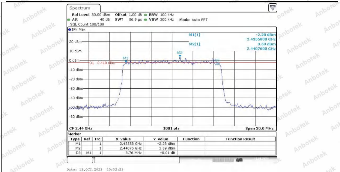
10M_Ant2_2440
