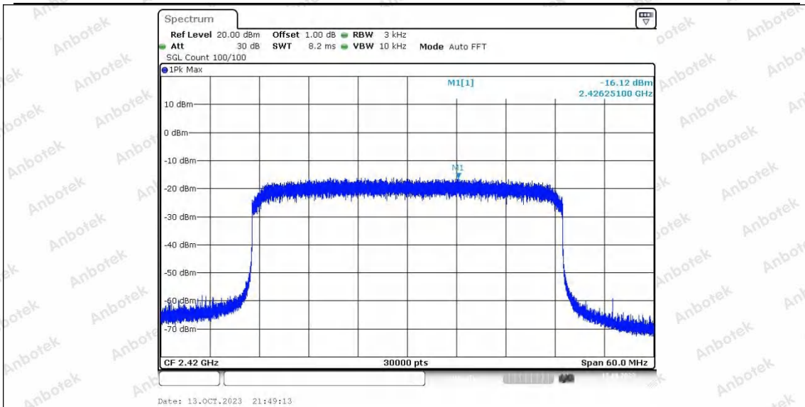
40M_Ant2_2420
