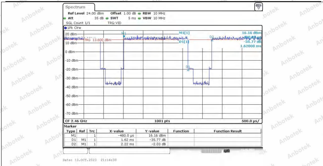
20M_Ant2_2460
