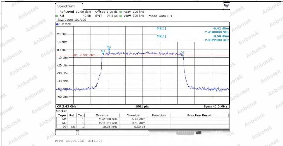
20M_Ant2_2420
