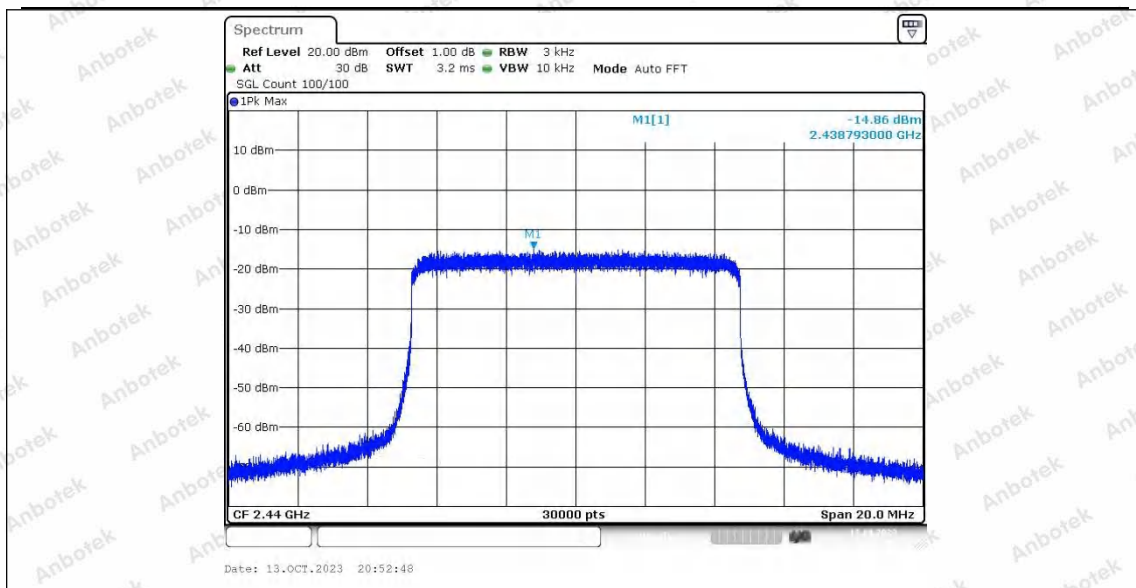
10M_Ant2_2440
