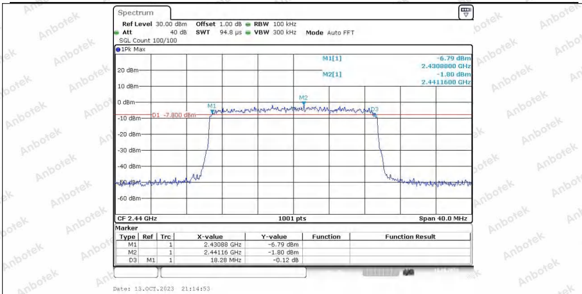
20M_Ant2_2440
