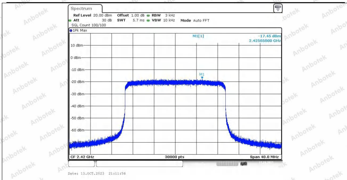
20M_Ant2_2420
