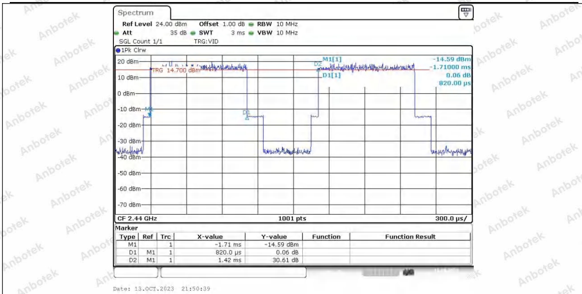
40M_Ant2_2440
