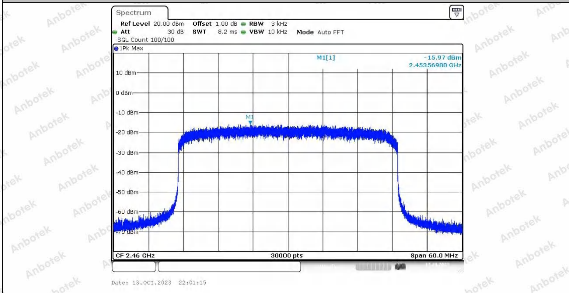
40M_Ant2_2460
