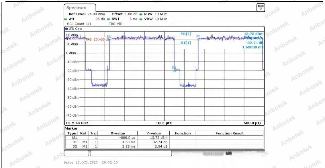
10M_Ant2_2440
