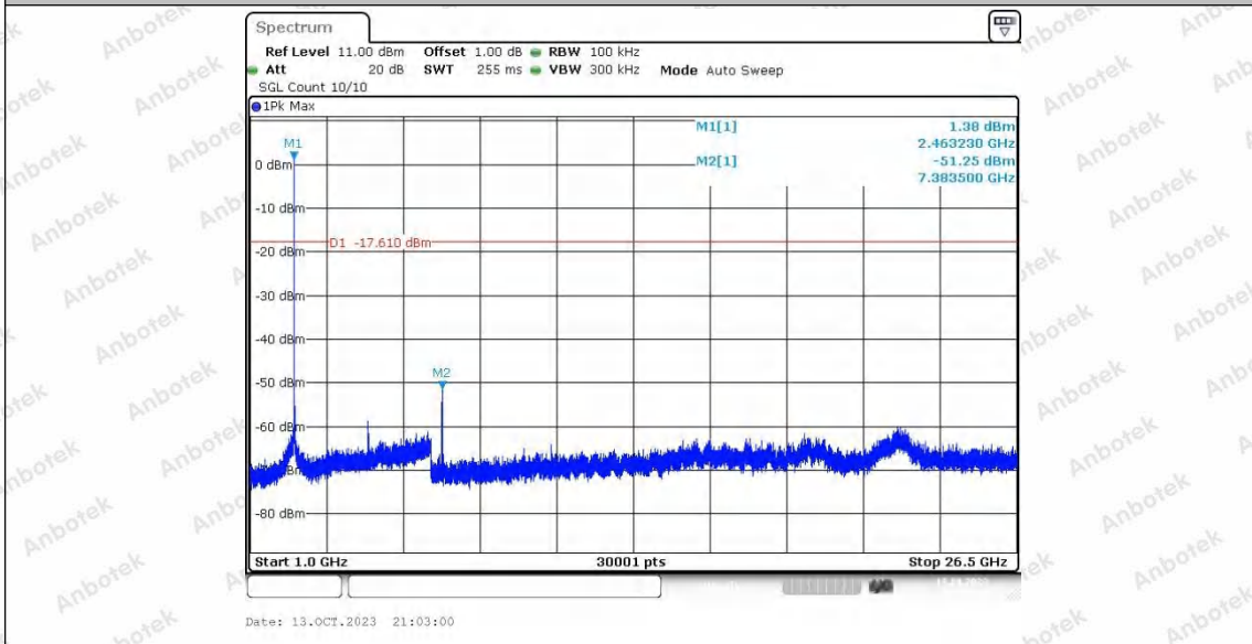
10M_Ant2_2460_1000~26500
