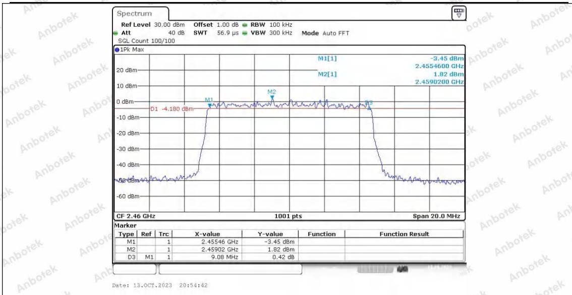
10M_Ant2_2460
