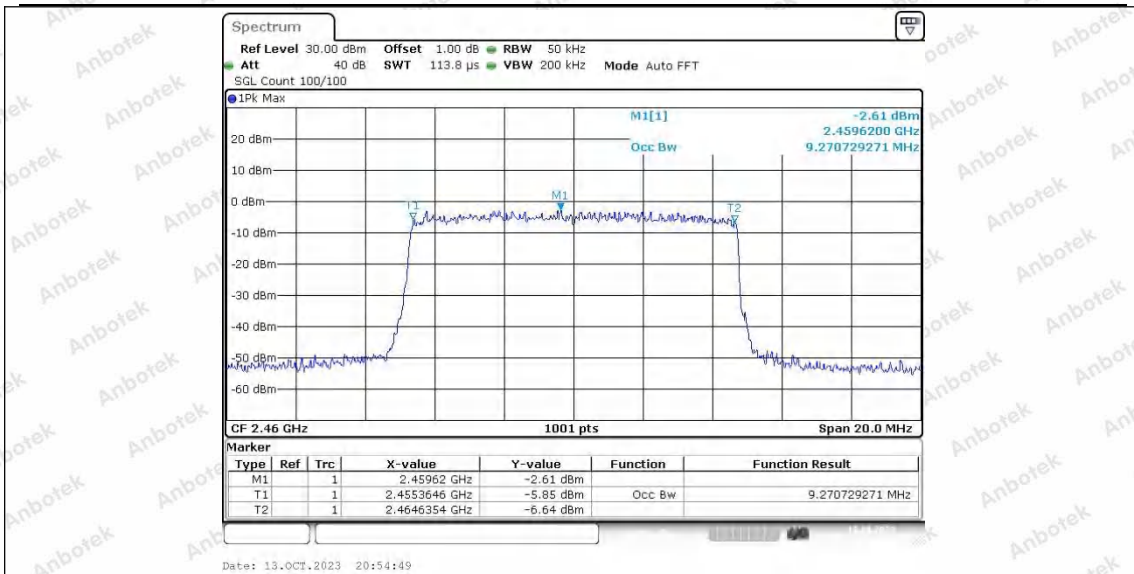
10M_Ant2_2460
