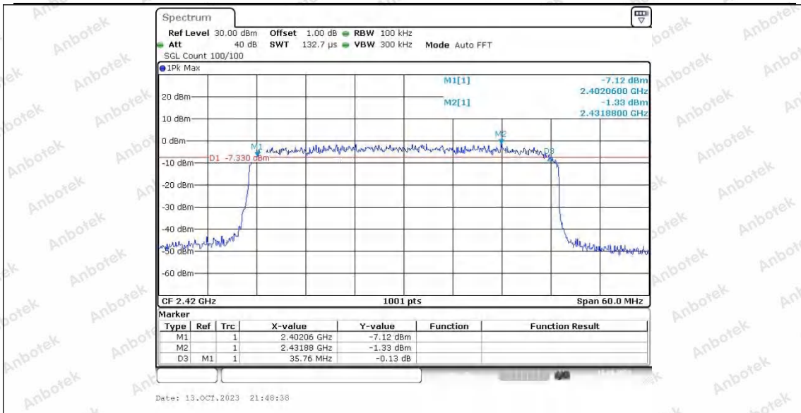
40M_Ant2_2420
