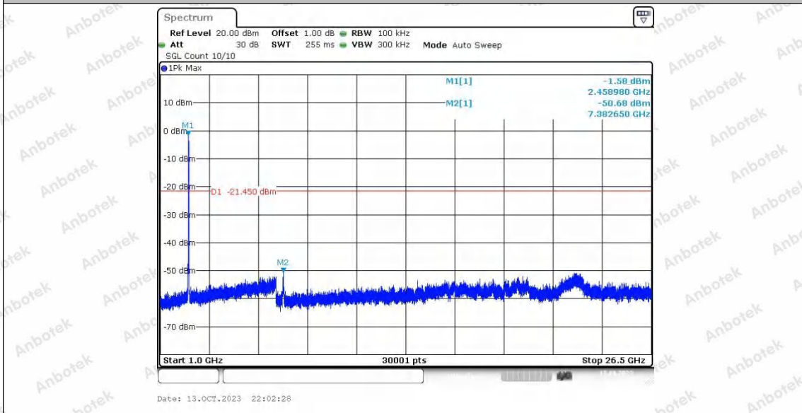
40M_Ant2_2460_1000~26500
