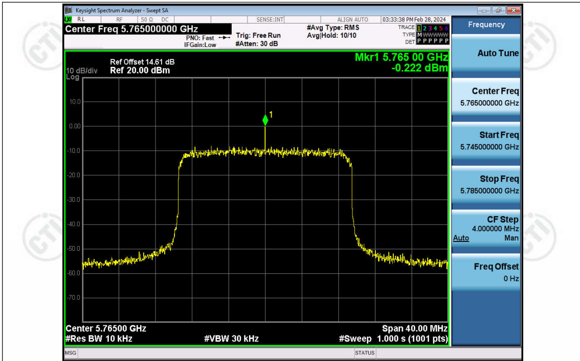
5G Slot 20MHz-Ant1-5765
