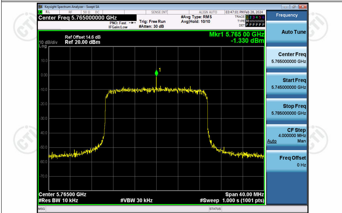
5G Slot 20MHz-Ant2-5765
