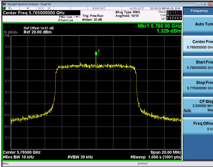
5G Slot 10MHz-Ant1-5765
