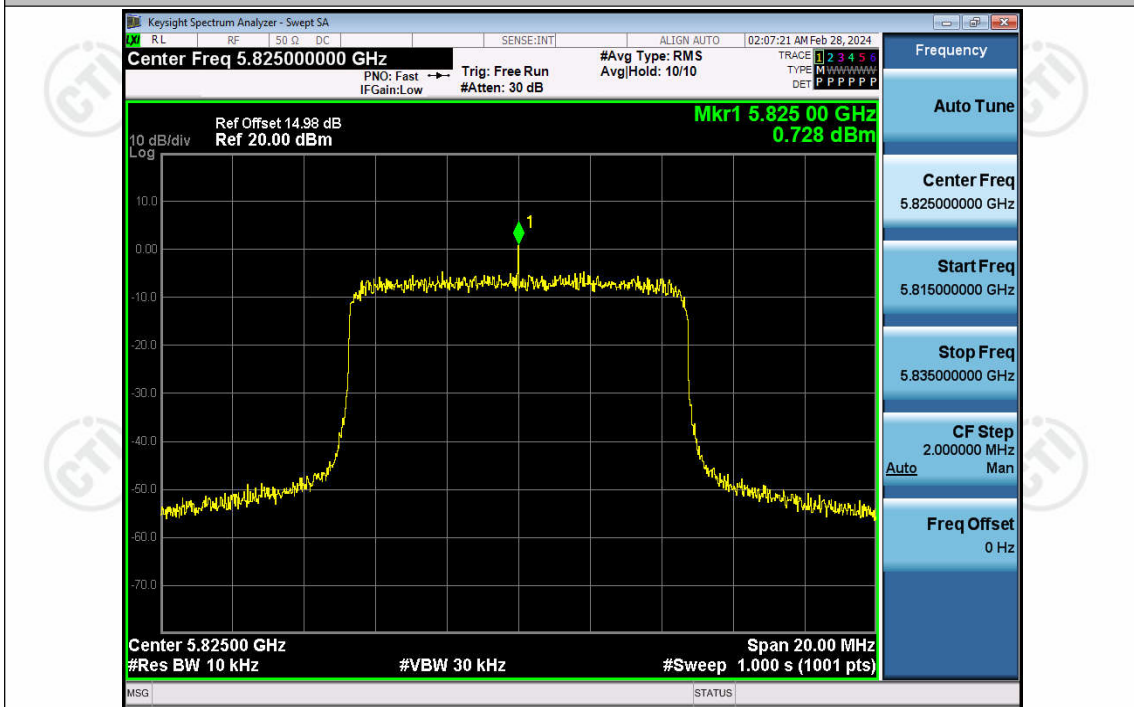
5G Slot 10MHz-Ant1-5825
