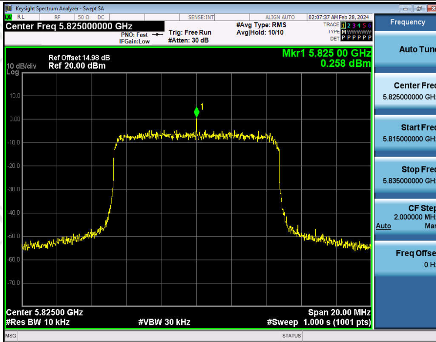
5G Slot 10MHz-Ant1-5825
