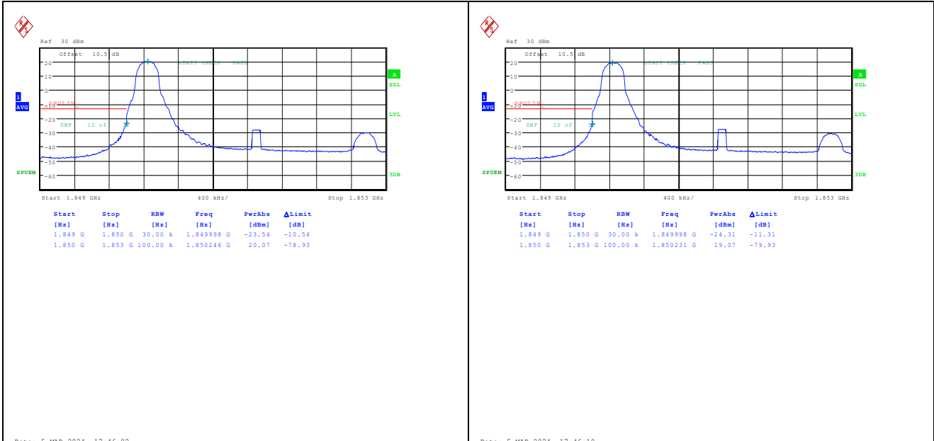
Band2_3MHz_QPSK_18615_1RB#0
