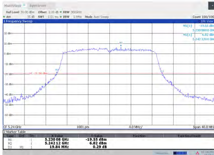
11ac20MIMO_Ant2_5240
