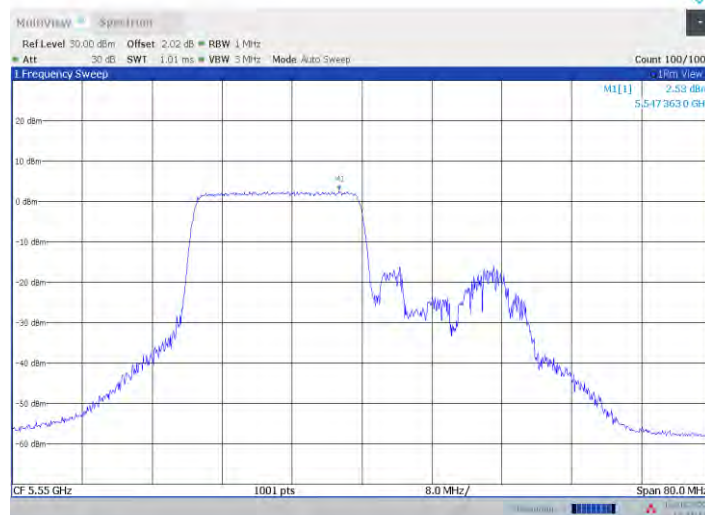
11ax40MIMO Ant2 5550 242Tone RU61
