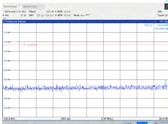
Band42-20MHz-QPSK-42190-1RB#0-Range2:0.15~30MHz
