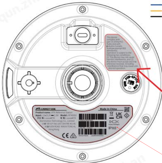
粘贴示意
