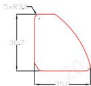
刀模图
