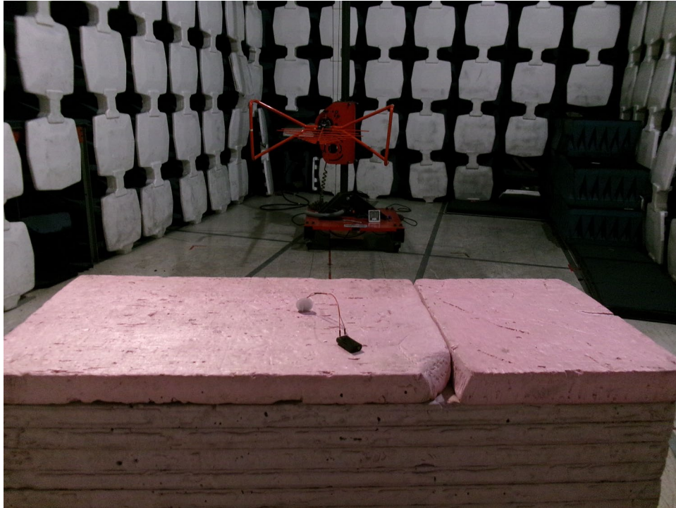
30-1000MHz
