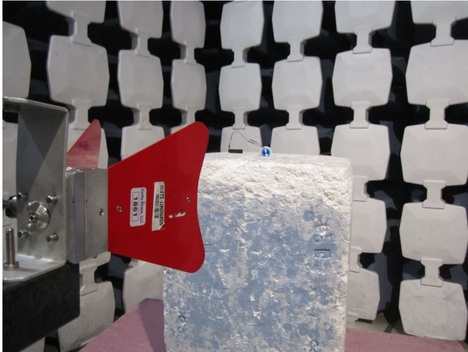
6-18GHz
