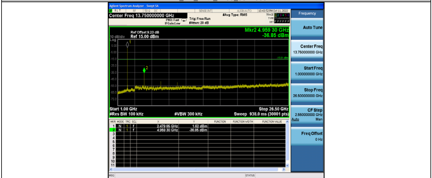
BLE_2M_Ant1_2480_1000~26500
