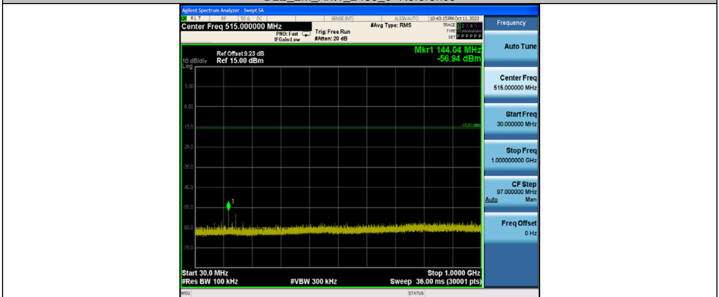
BLE_2M_Ant1_2480_30~1000
