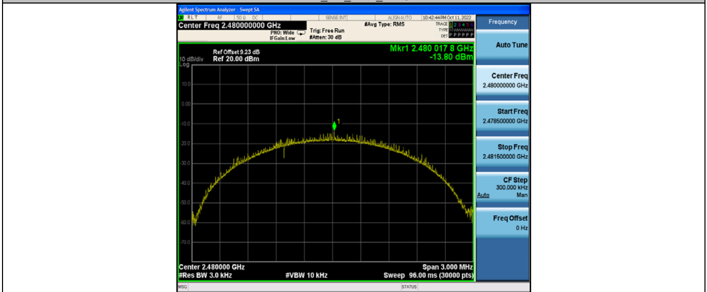
BLE_2M_Ant1_2480
