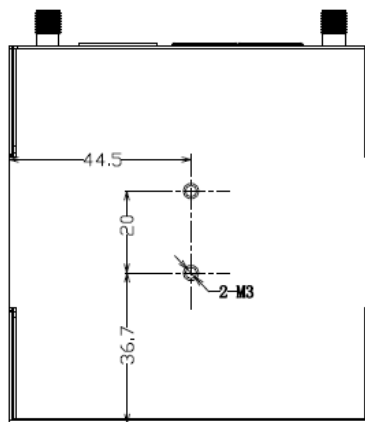
DIN Rail installing position
