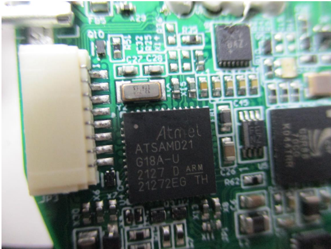
BT Module
