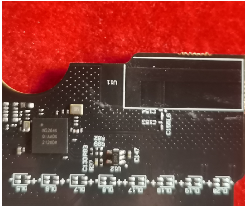
BLE chip & antenna
