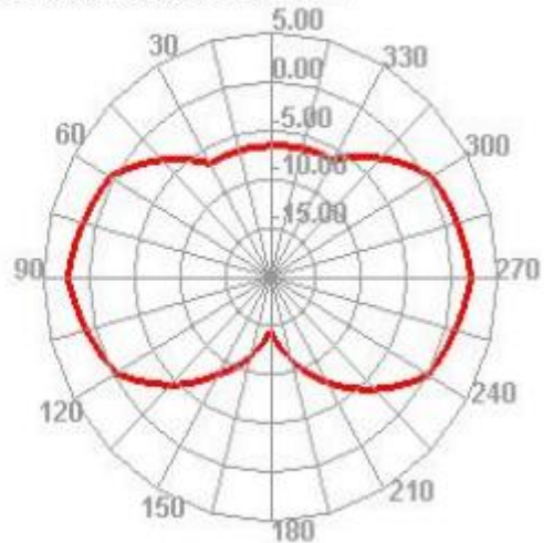
2450.000MHz E2
