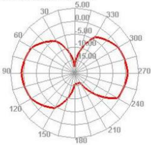
2400.000MHz E1
