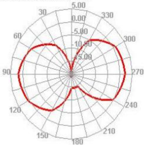
2450.000MHz E1
