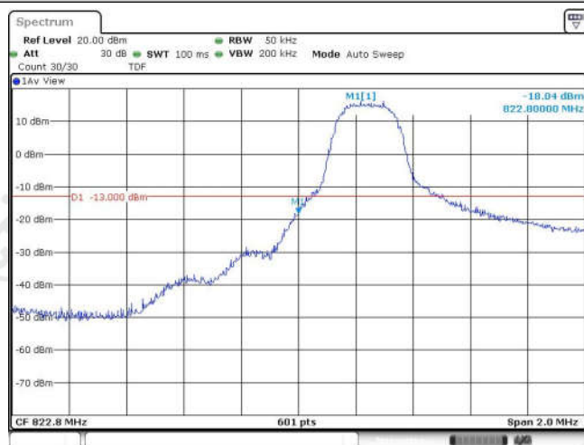
Band26-3MHz-QPSK-26793-1RB#0
