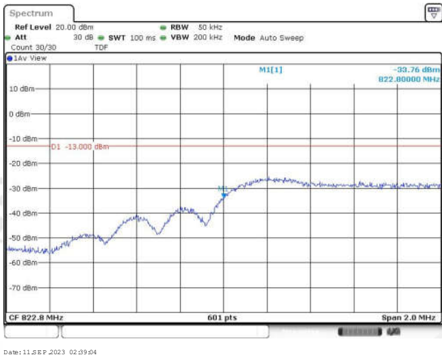
Band26-3MHz-QPSK-26793-15RB#0
