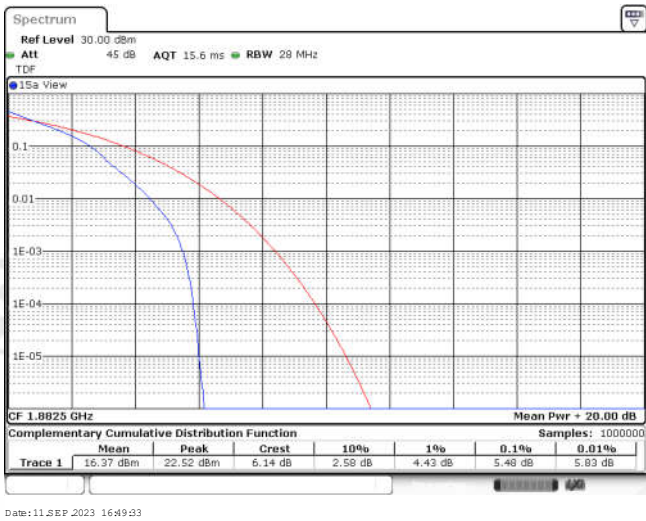
Band25-10MHz-QPSK-26365-50RB#0
