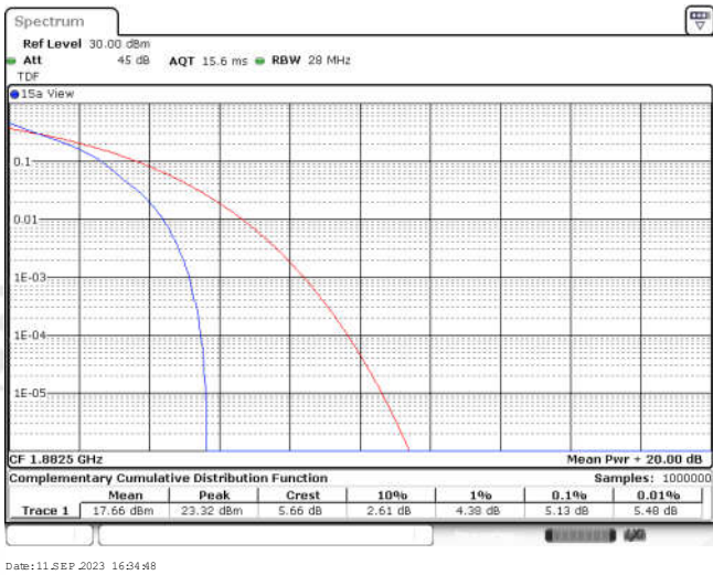
Band25-3MHz-QPSK-26365-15RB#0
