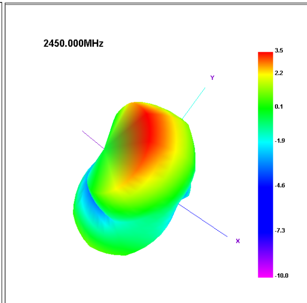
2450MHz
