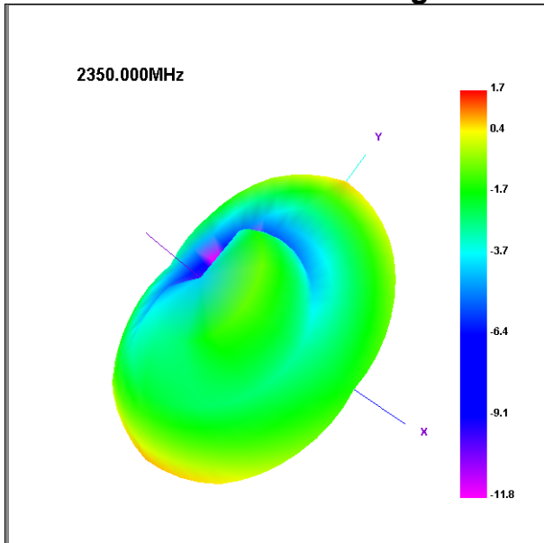
2350MHz
