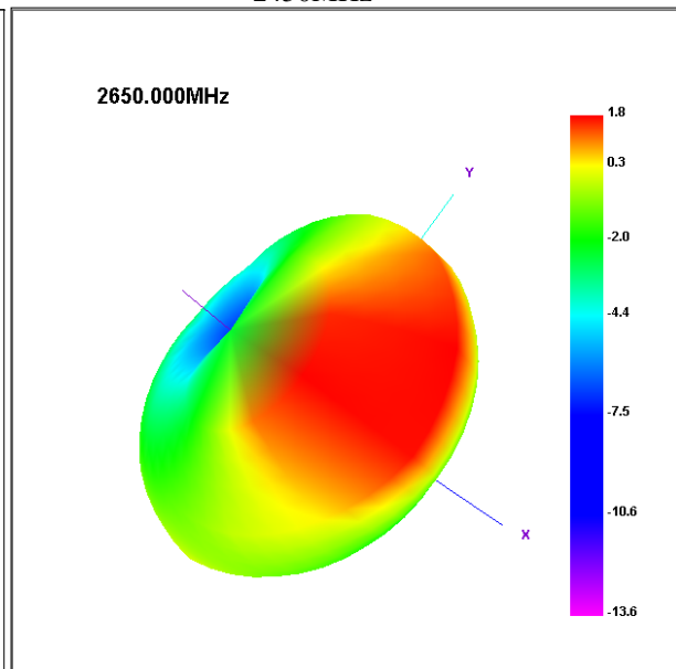
2650MHz
