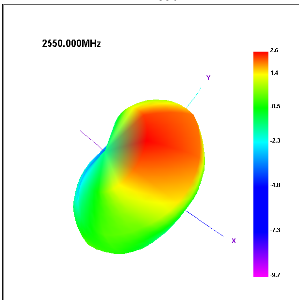
2550MHz
