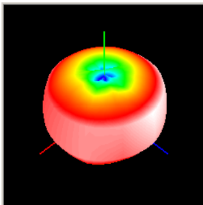
6 GHz z
