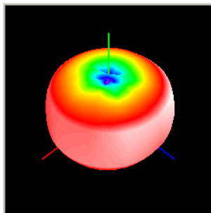
2.45 GHz z
