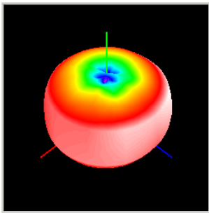
5GHz z
