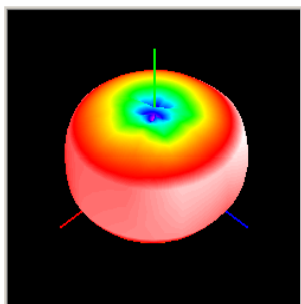
2.4 GHz z
