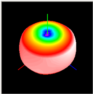
5.5 GHz z
