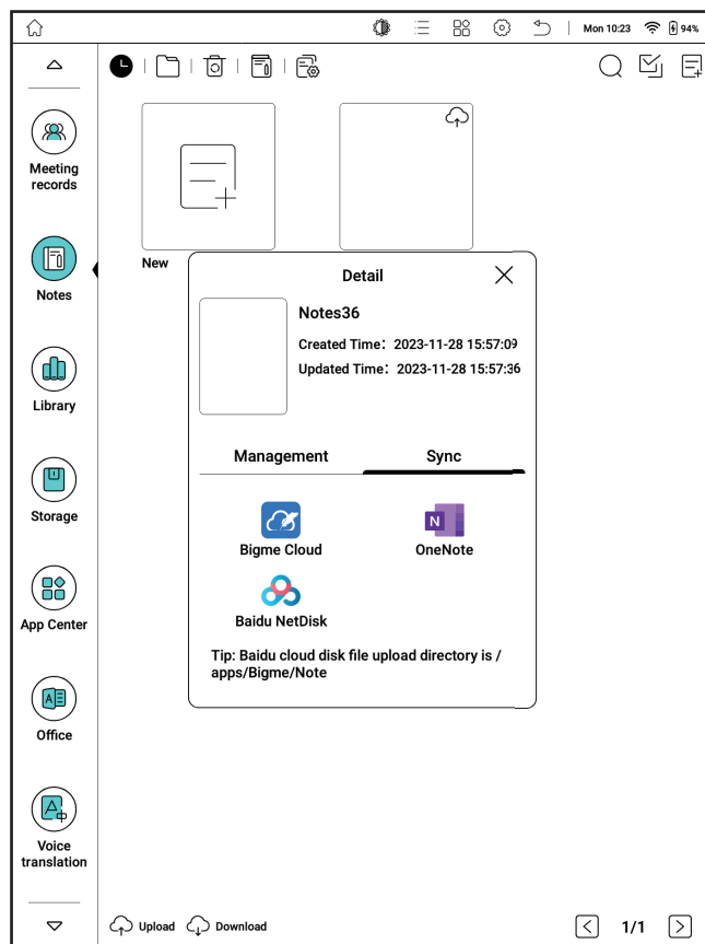
Long Press
