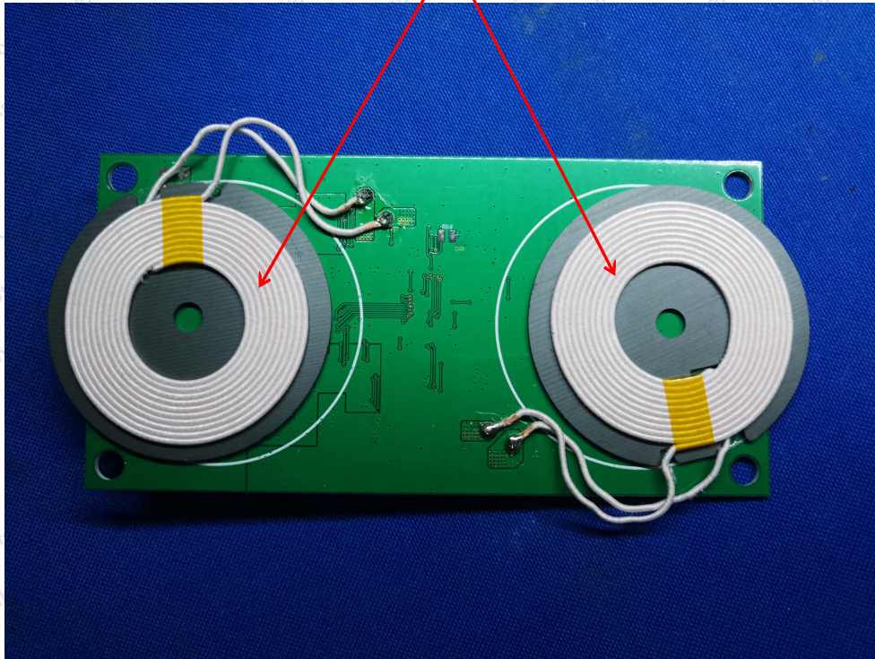
WPT ANT
