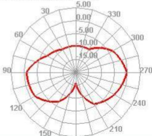
5100.000MHz E2
