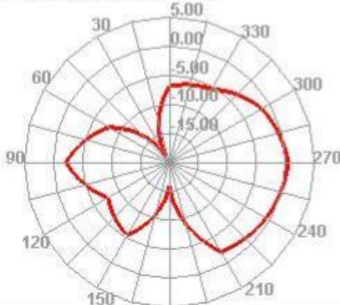
5100.000MHz E1
