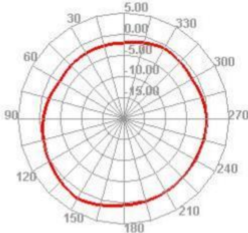
5100.000MHz H
