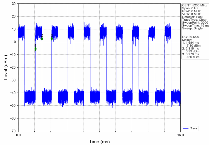
802.11n(HT40)_HCH_5230MHz_Ant1_NTNV
