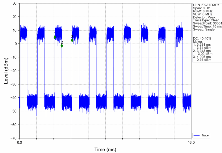
802.11ac(VHT40)_HCH_5230MHz_Ant1_NTNV
