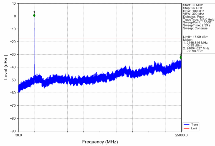
802.11n(HT40) MCH_2437MHz_Ant2 (MIMO) NTN
