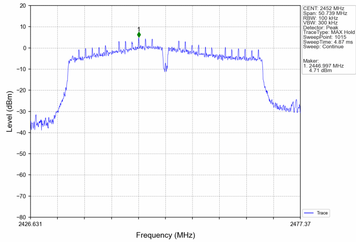
802.11n(HT40) HCH_2452MHz_Ant2 (MIMO) NTVN
