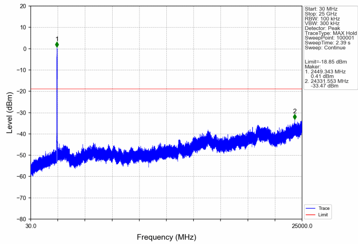
802.11n(HT40) HCH_2452MHz_Ant2 (MIMO) NTNV
