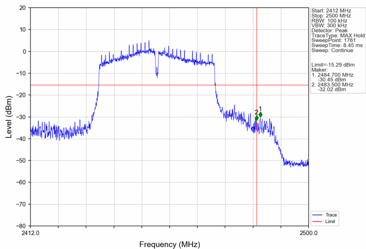
802.11n(HT40) HCH_2452MHz_Ant1 (MIMO) NTNV
