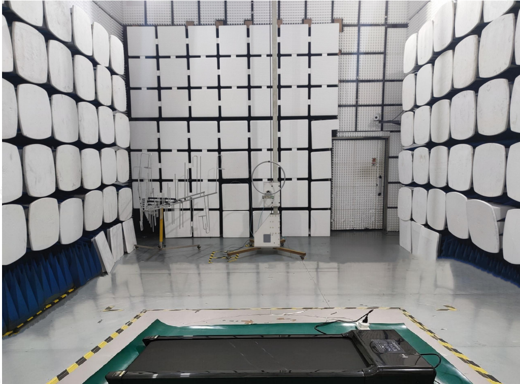
Fig. 1 (Below 30MHz)
