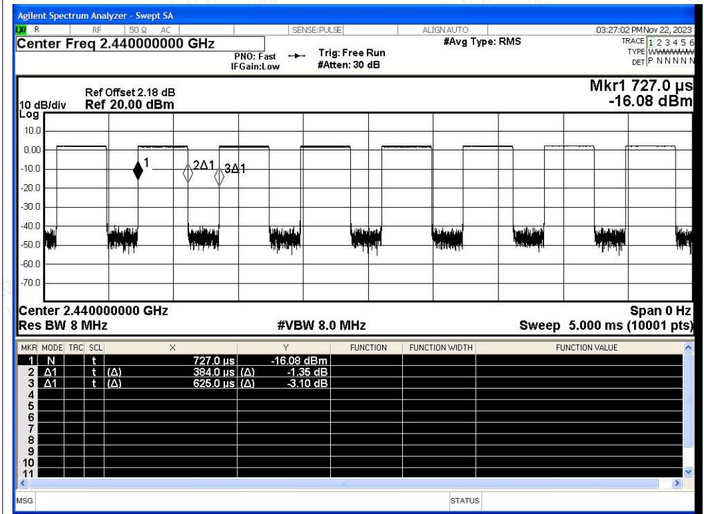
Duty Cycle NVNT BLE 1M 2440MHz Ant1
