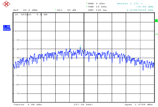
High -19.66dBm/3kHz
