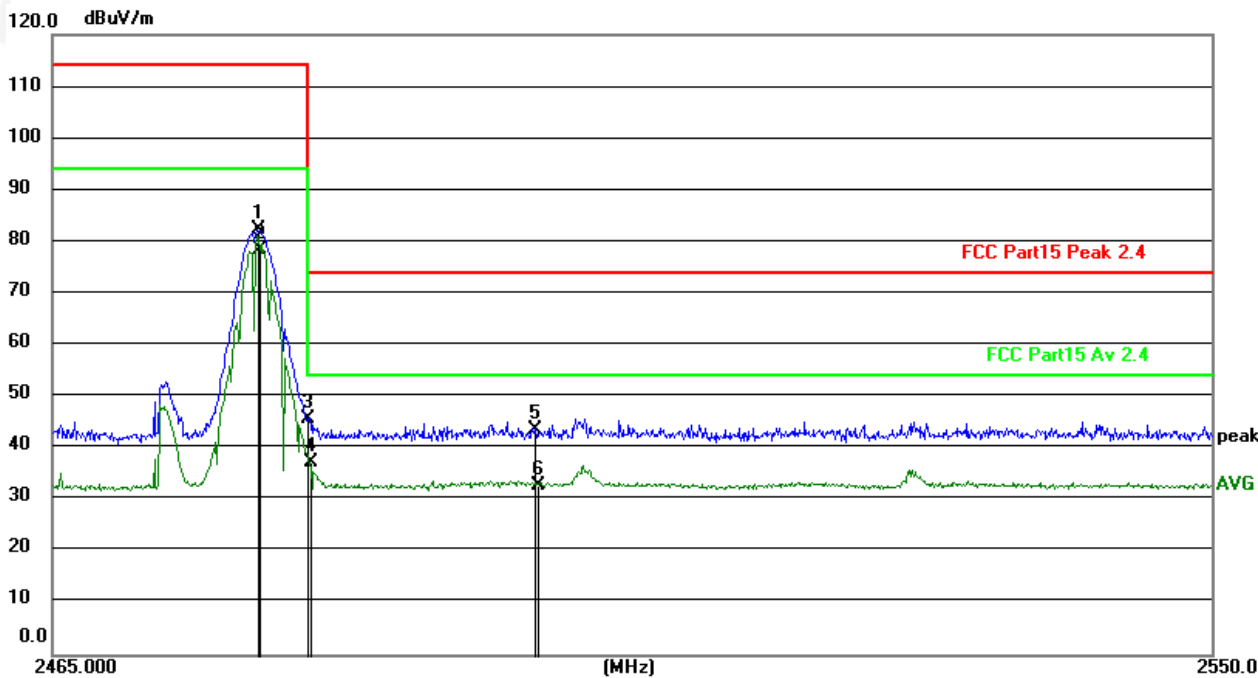
2480MHz Horizontal
