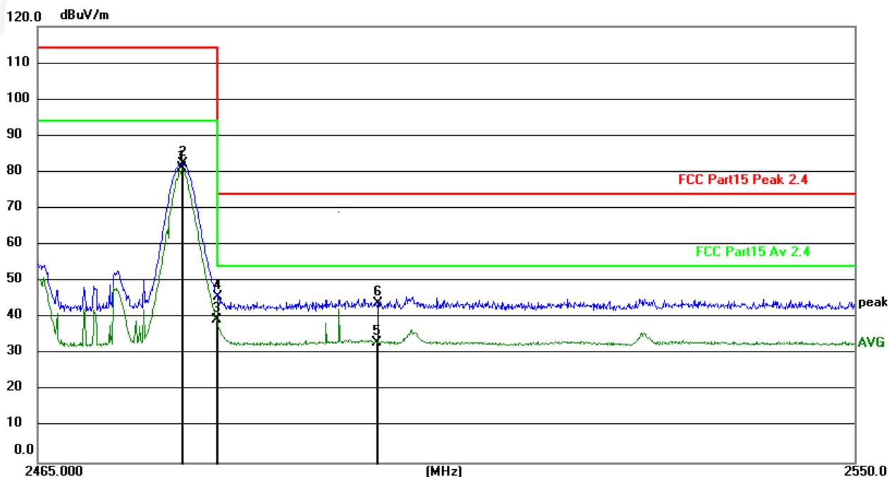
2480MHz Horizontal
