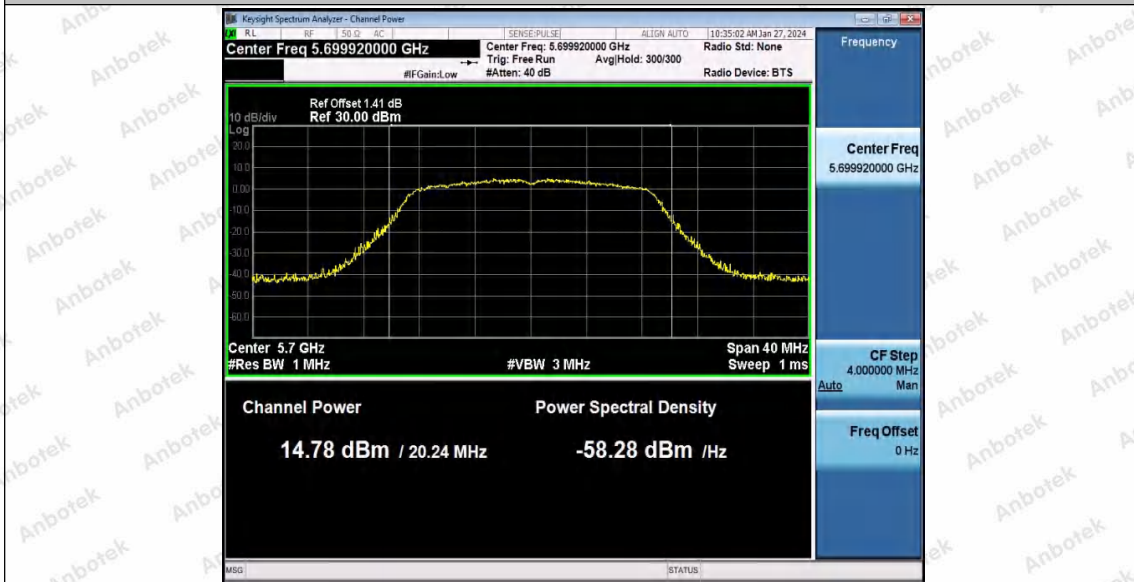
802.11n(HT20) SISO_Ant1_5700
