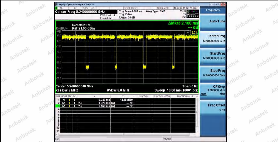
802.11n(HT20) SISO_Ant1_5240
