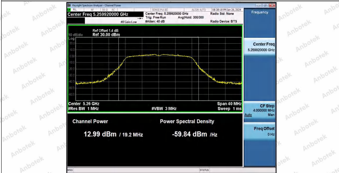
802.11a_Ant1_5260
