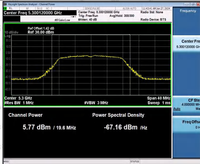
802.11a_Ant1_5300
