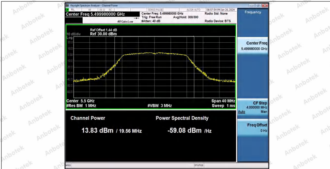
802.11a_Ant1_5500
