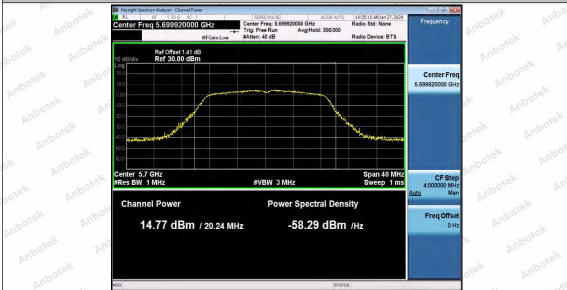
802.11n(HT20) SISO_Ant1_5700
