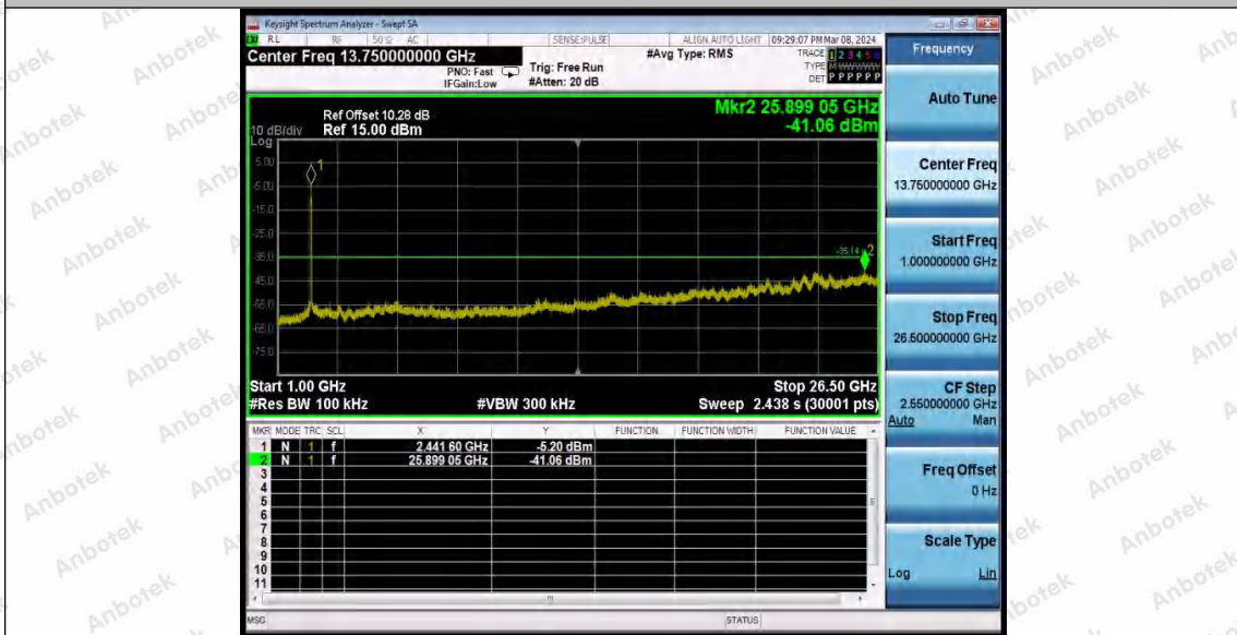
802.11n(HT40) SISO_Ant1_2452_0~Reference
