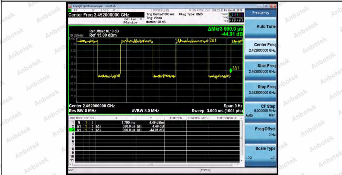
802.11n(HT40) SISO_Ant1_2452
